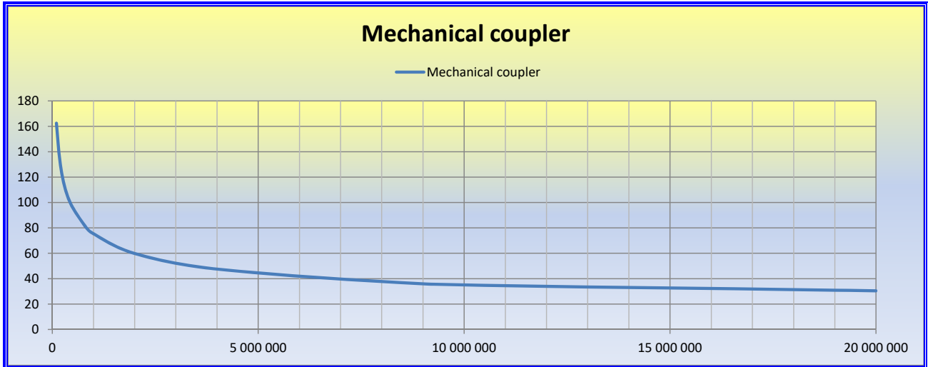
Figure 2 : Forme de la courbe caractéristique de résistance en fatigue d'un raboutage mécanique selon EUROCODE 2
