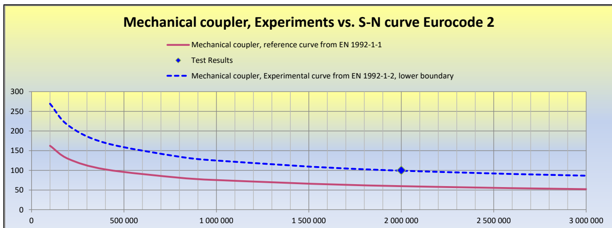
Figure 3 : Exemple avec une valeur de \Delta\sigma applicable à deux millions de cycles égale à 100 MPa
