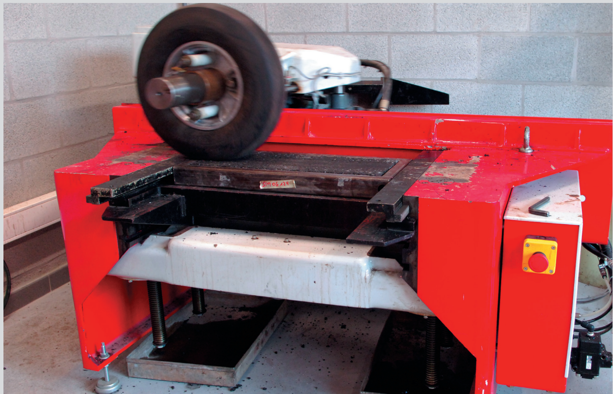
← Compacteur de plaques. © SPW-Direction de l'Édition
