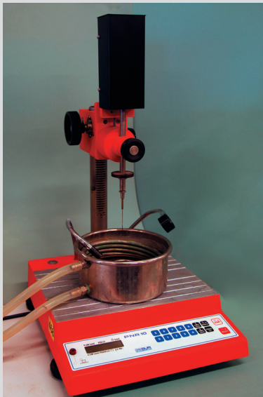
Bain thermostatique et pénétromètre à aiguille. © SPW-Direction de l'Édition
