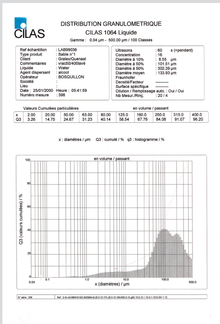
← Exemple d'expression des résultats avec diagramme. © SPW-Direction de la Recherche et du Contrôle routier
