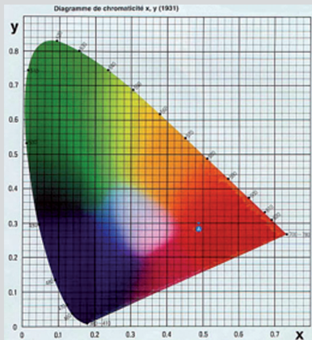
Diagramme de chromaticité © SPW-Direction de la Recherche et du Contrôle routier
