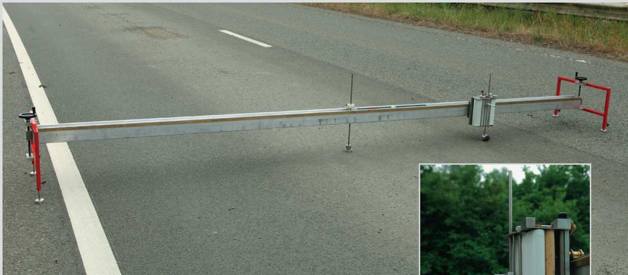
Le transversoprofilographe. © SPW-Direction de l'Édition
