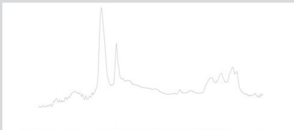
Spectre FTIR d'un bitume routier © SPW-Direction de la Recherche et du Contrôle routier
