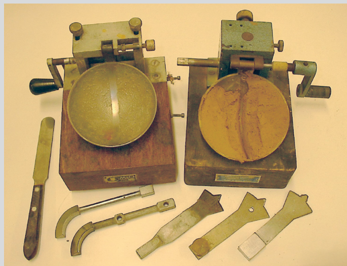
Appareil de Casagrande (limite de liquidité). © SPW-Direction de la Recherche et du Contrôle routier
