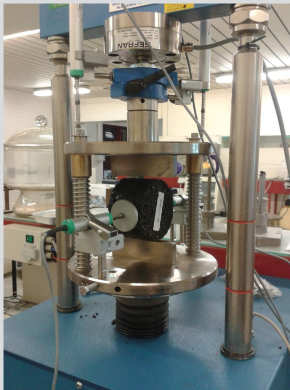
← Presse permettant de déterminer la résistance à la traction indirecte © SPW-Direction de l'Édition
